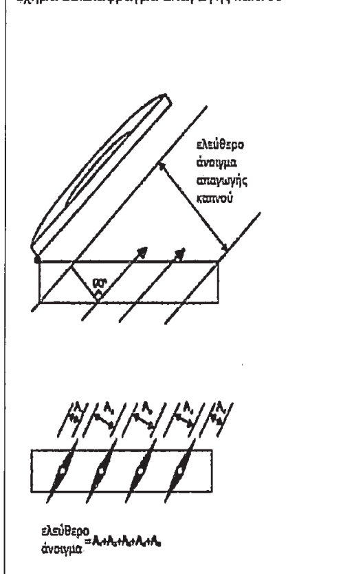
Σχήμα 22: Διάφραγμα απαγωγής καπνού
